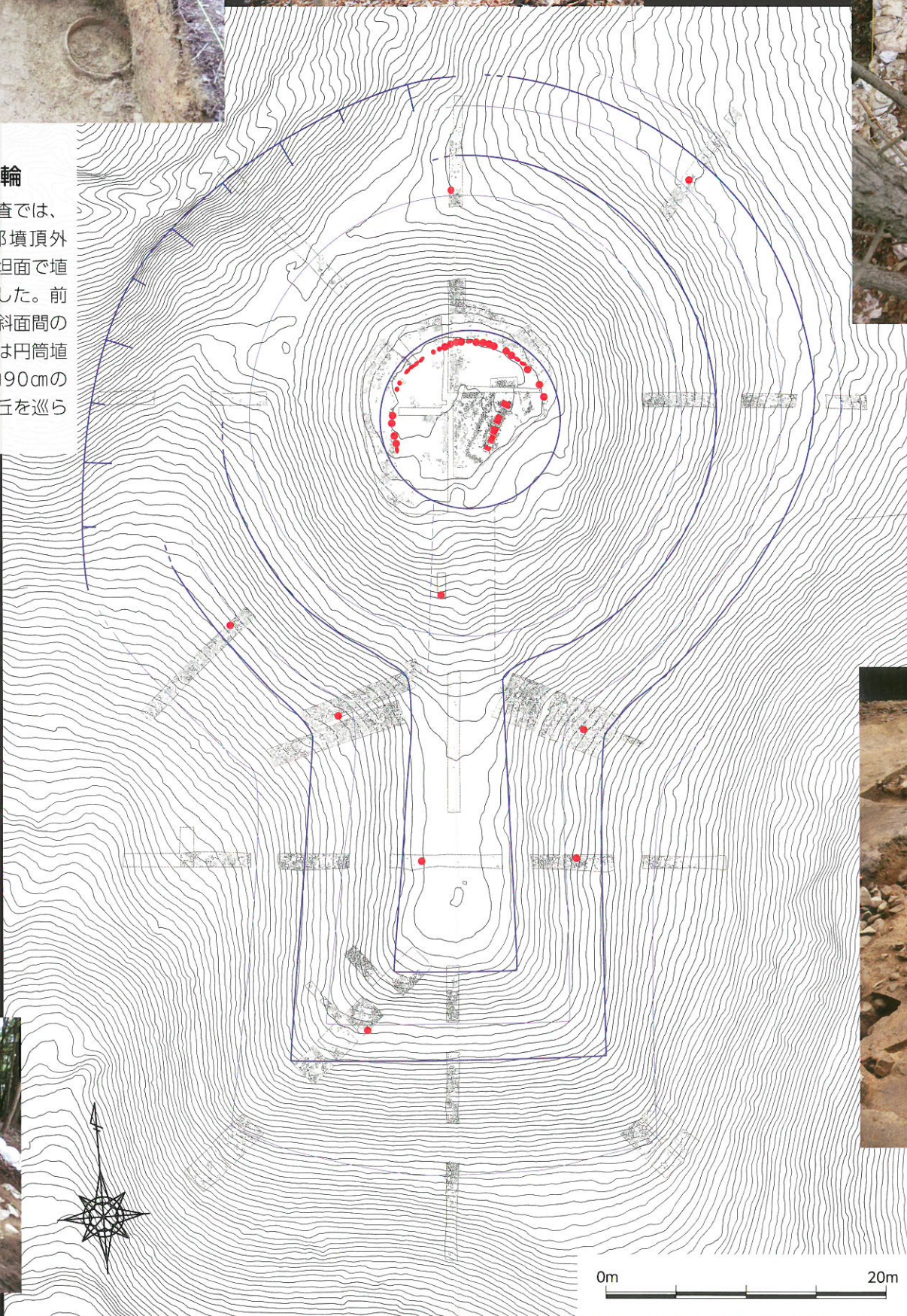
墳丘測量図
